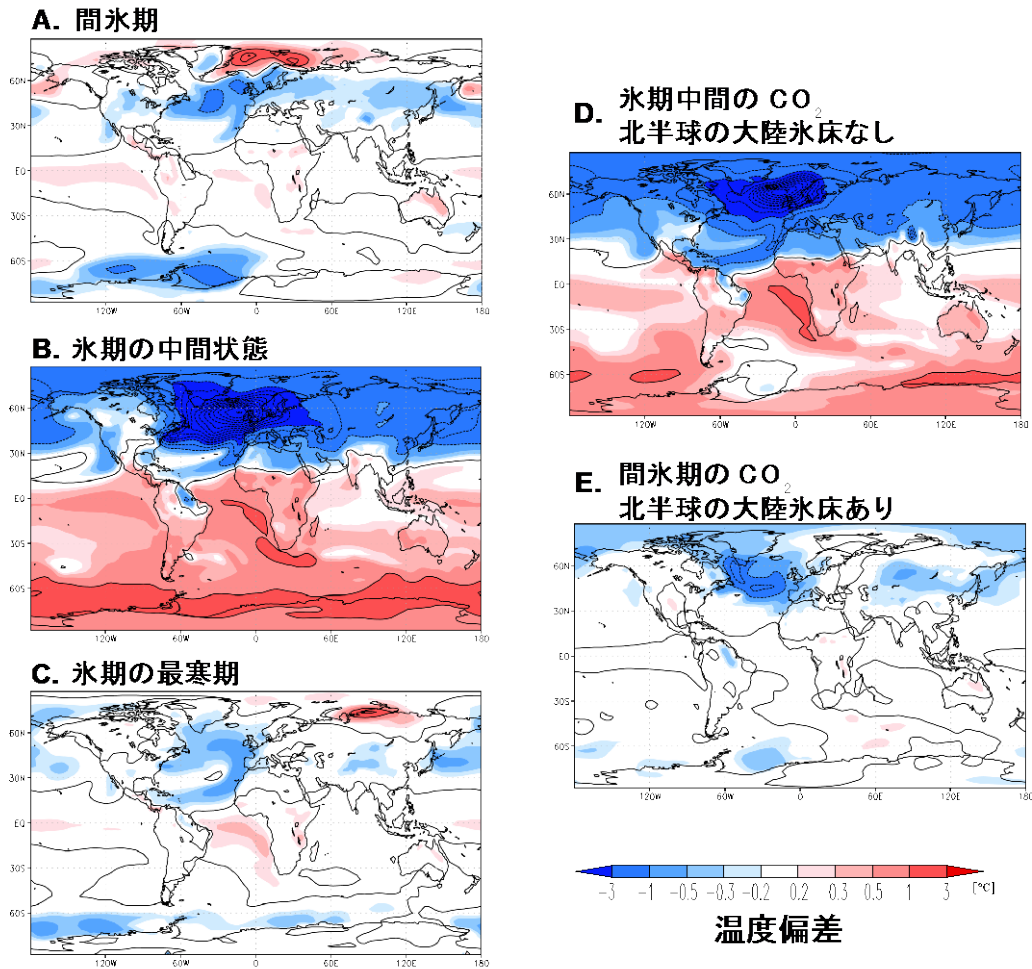
図 4：大気海洋結合大循環モデル (MIROC) による気候シミュレーションの結果。(A-C) まず3つの異なる気候状態を再現した(間氷期、氷期の中間状態、氷期最寒期のそれぞれに相当する大気中二酸化炭素濃度と氷床形状を与えた)。その後、北大西洋北部に淡水を500年間加え続けた後の初期状態からの温度偏差を示す。氷期の中間状態の時に反応が大きく、北半球が寒冷化し、南半球は逆に温暖化することが分かる。(D, E) 現実には存在しなかった条件下での感度実験の結果。間氷期の条件から、大気中二酸化炭素濃度または北半球氷床のみを氷期の中間状態と同じにした。その結果、気候の不安定性が増大する要因として大気中二酸化炭素の役割が大きかった。
